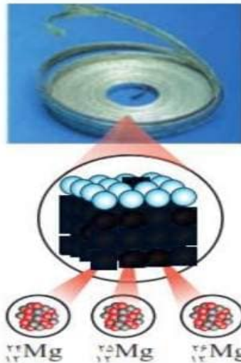
ایزوتوپهای منیزیم
