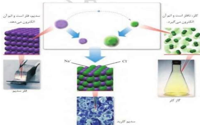
شکل ۲۵- واکنش اتم های سدیم با کلر، دادوستد الکترون و تشکیل سدیم کلرید
